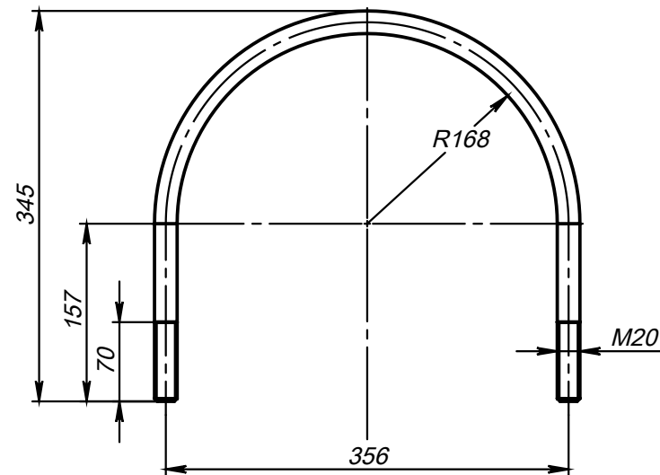
Поз.6 (Хомут)
