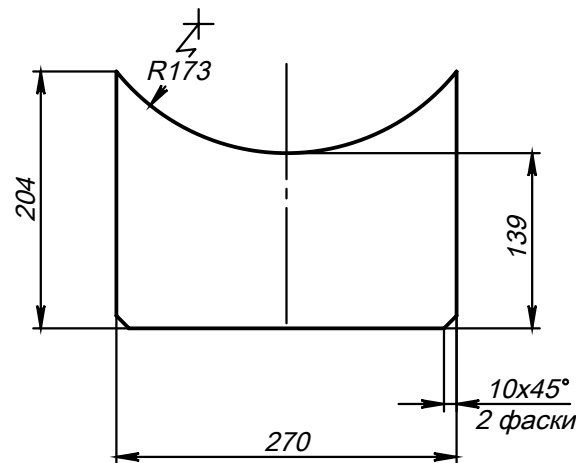
Поз.2 (Ребро)
