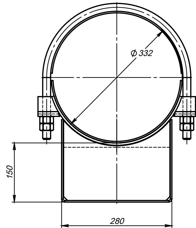
Поз.4 (Ложмент)
