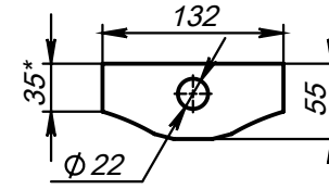
Поз.5 (Ушко) развертка
