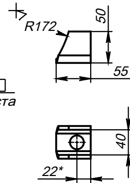
Поз.5 (Ушко)
