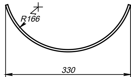
Поз.2 (Ребро)
