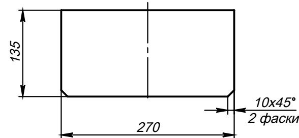
Поз.3 (Ребро среднее)
